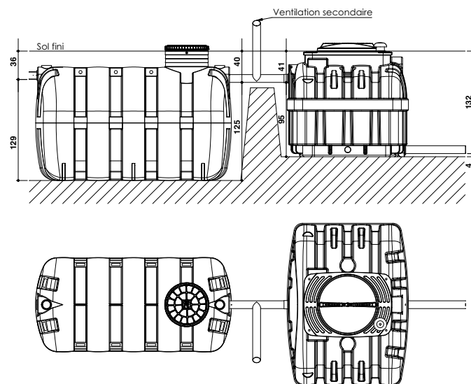
Filtre compact Biomeris 4 EH
